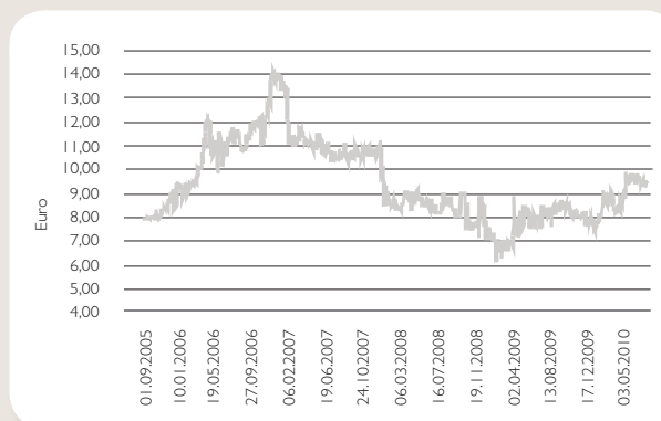
C-aktiens kursutveckling 1.9.2005–31.8.2010
